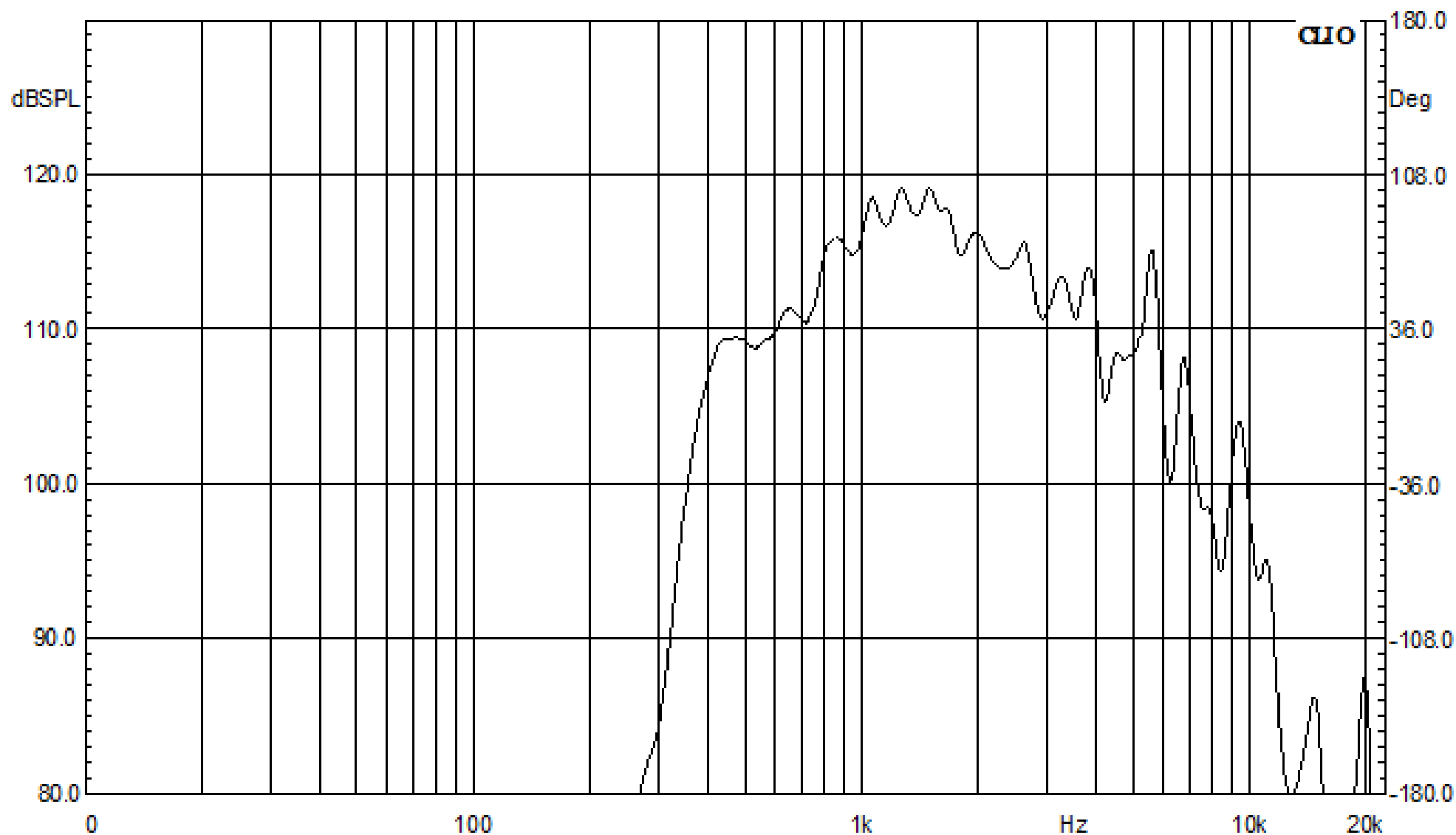
АЧХ RSH-15, 15Вт
